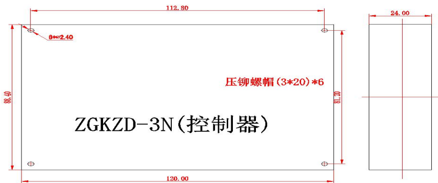
正视图
